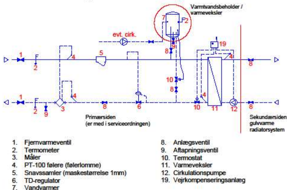
PRINCIPDIAGRAM AF ANLÆG Skitse gældende serviceordningen
