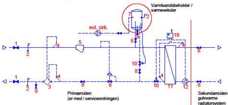
PRINCIPDIAGRAM AF ANLÆG Skitse gældende serviceordningen
